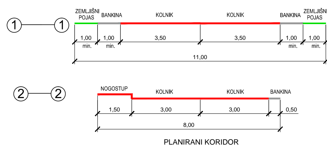
POPREČNI PROFIL M 1 : 100
